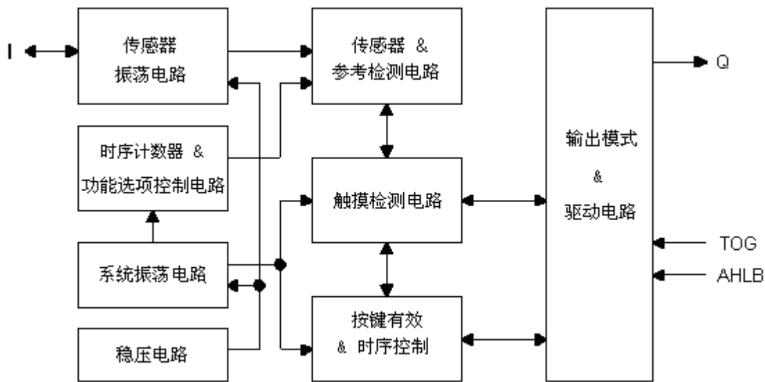
方块图
