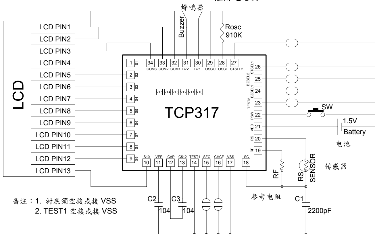
TCP317A/TCP317B 应用电路图
